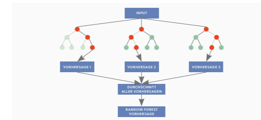
Abb.: Random Forest mit numerischen Variablen
