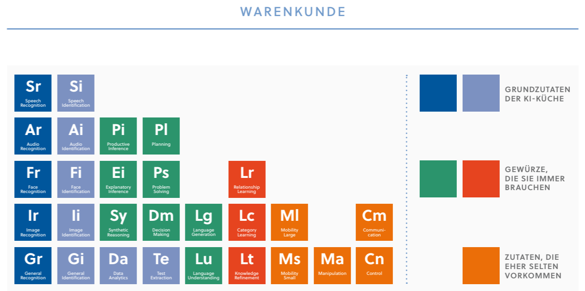
Abbildung 8: KI-Periodensystem
